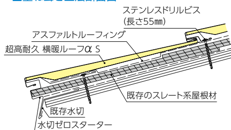
■重ね葺き工法断面図
